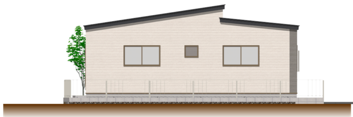
● 北側 立面図
